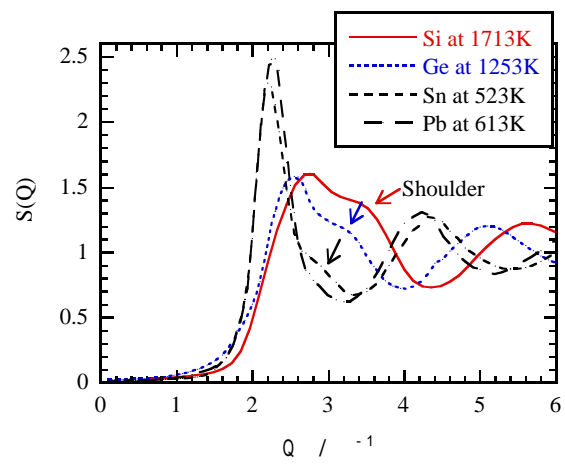
図7. 14(IVb)族液体の融点近傍における構造因子
