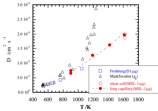
図5 . 液体Snの自己拡散係数
