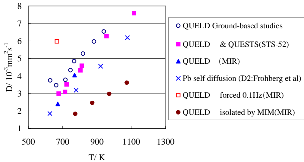
図4. Pb中の不純物Au拡散係数に及ぼすg-ジッタ-の影響 (カナダMIM)
